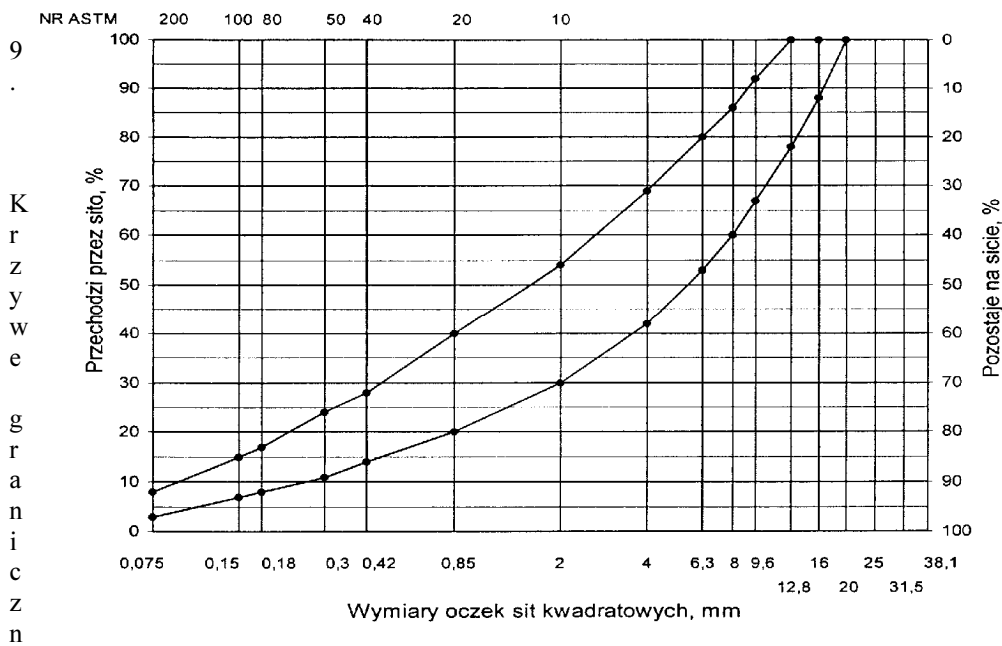
e uziarnienia mieszanki mineralnej BA od 0 do 16 mm do warstwy wiążącej, wyrównawczej i wzmacniającej nawierzchni drogi o obciążeniu ruchem KR1 lub KR2
