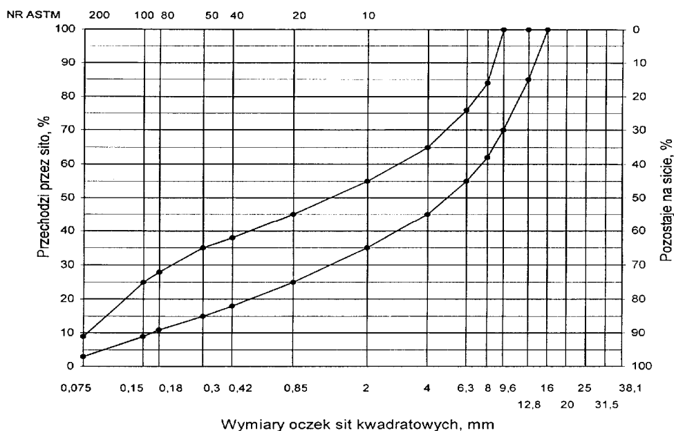
Rys. 10. Krzywe graniczne uziarnienia mieszanki mineralnej BA od 0 do 12,8 mm do warstwy wiążącej, wyrównawczej i wzmacniającej nawierzchni drogi o obciążeniu
