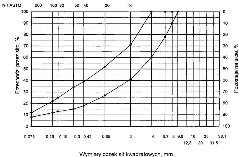
Rys. 2. Krzywe graniczne uziarnienia mieszanki mineralnej BA od 0 do 8mm, od 0 do 6,3 mm do warstwy ścieralnej nawierzchni drogi o obciążeniu w ruchu nawierzchni
